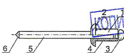
Рис.1. Общий вид заклепки
