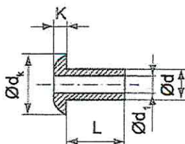
Рис. 3. Геометрические параметры гильзы заклепки
